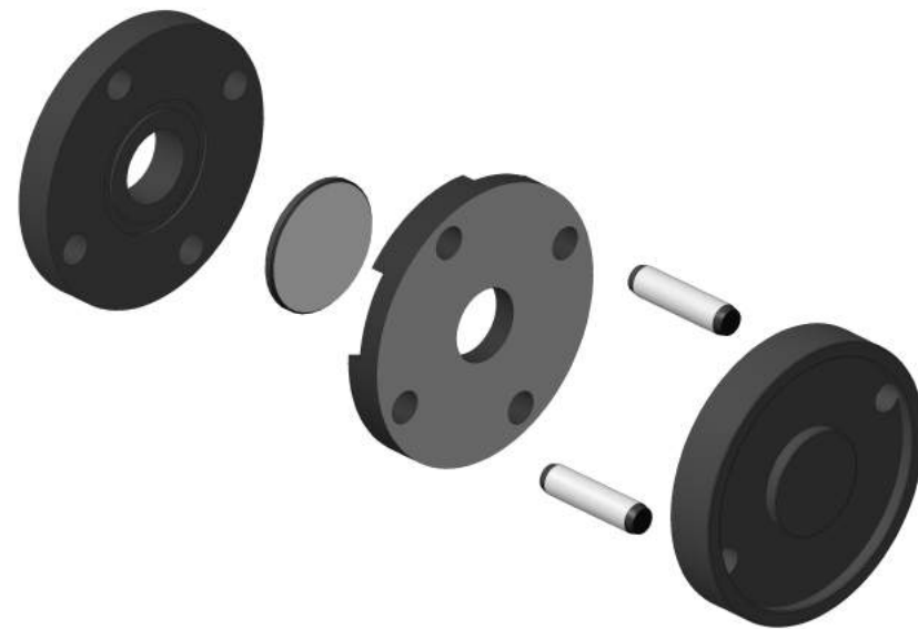
порядок сборки
